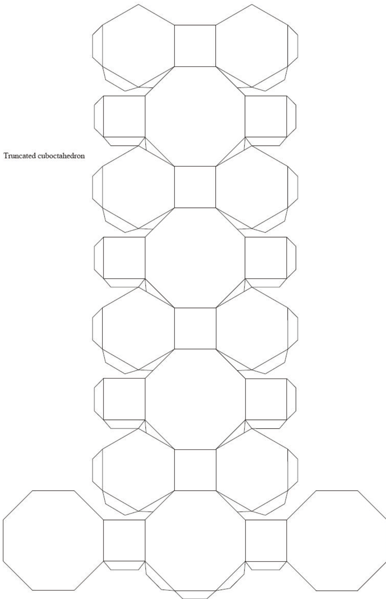
Gran rombicuboctaedre
